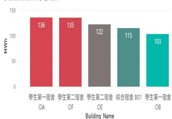
學生宿舍各棟用電比較
